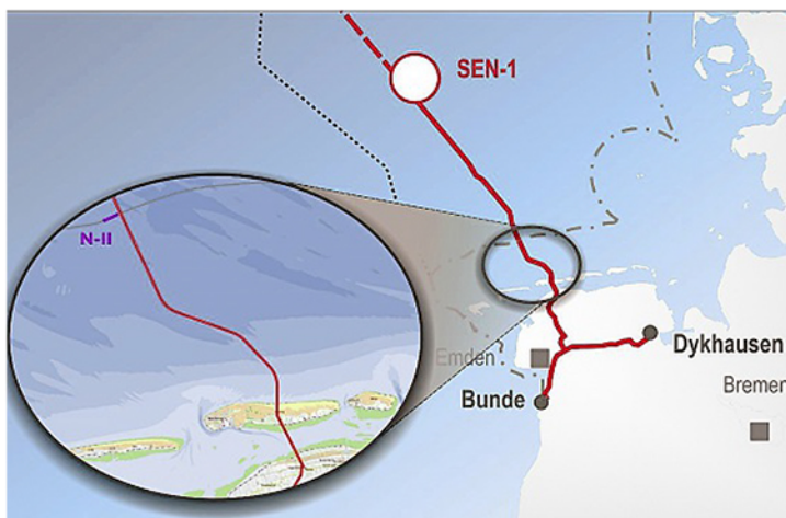
Möglicher Verlauf einer Wasserstoffpipeline an der Nordseeküste.
